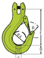
Gancho para cadena con lengüeta de seguridad for jada - grado 100
