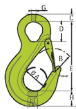
Gancho de anilla con lengüeta de seguridad for jada - grado 100
