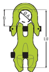
Acortador de cadena con "U link" y "seguridad"- grado 100
